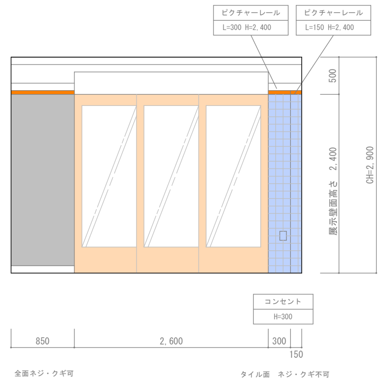
展開図 d S = 1 / 50
