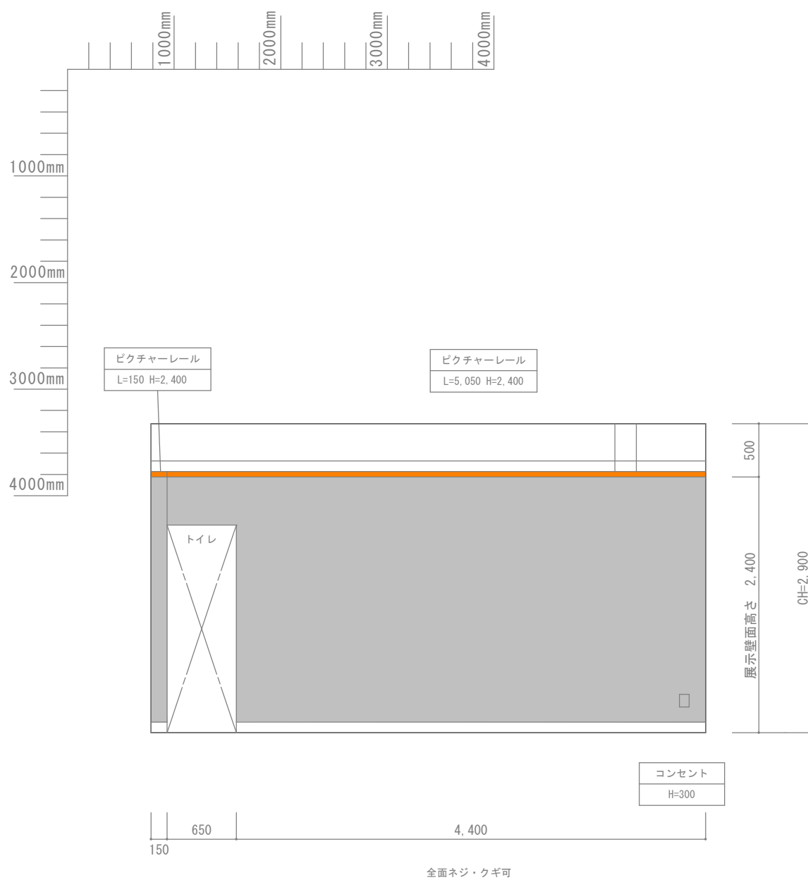
展開図 c S = 1 / 50
